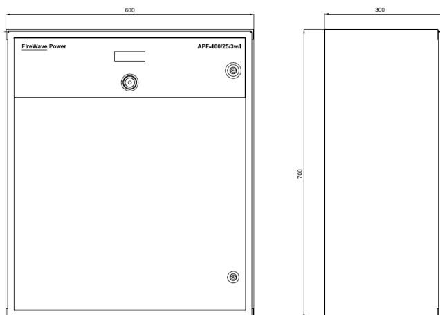
APF-100/25/3w/I – rysunek katalogowy
