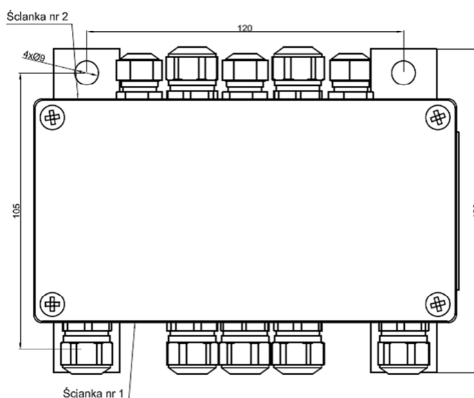
Skrzynka rozgałęźna typu SR-03/523/* – rysunek katalogowy
