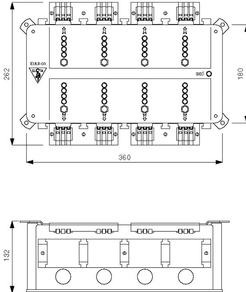
URZĄDZENIE DO ŁADOWANIA BATERII TYPU EULB-03 – rysunek katalogowy
