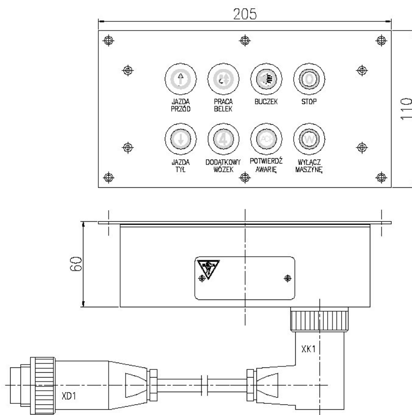
KLAWIATURA TYPU EKMS-01 – rysunek katalogowy
