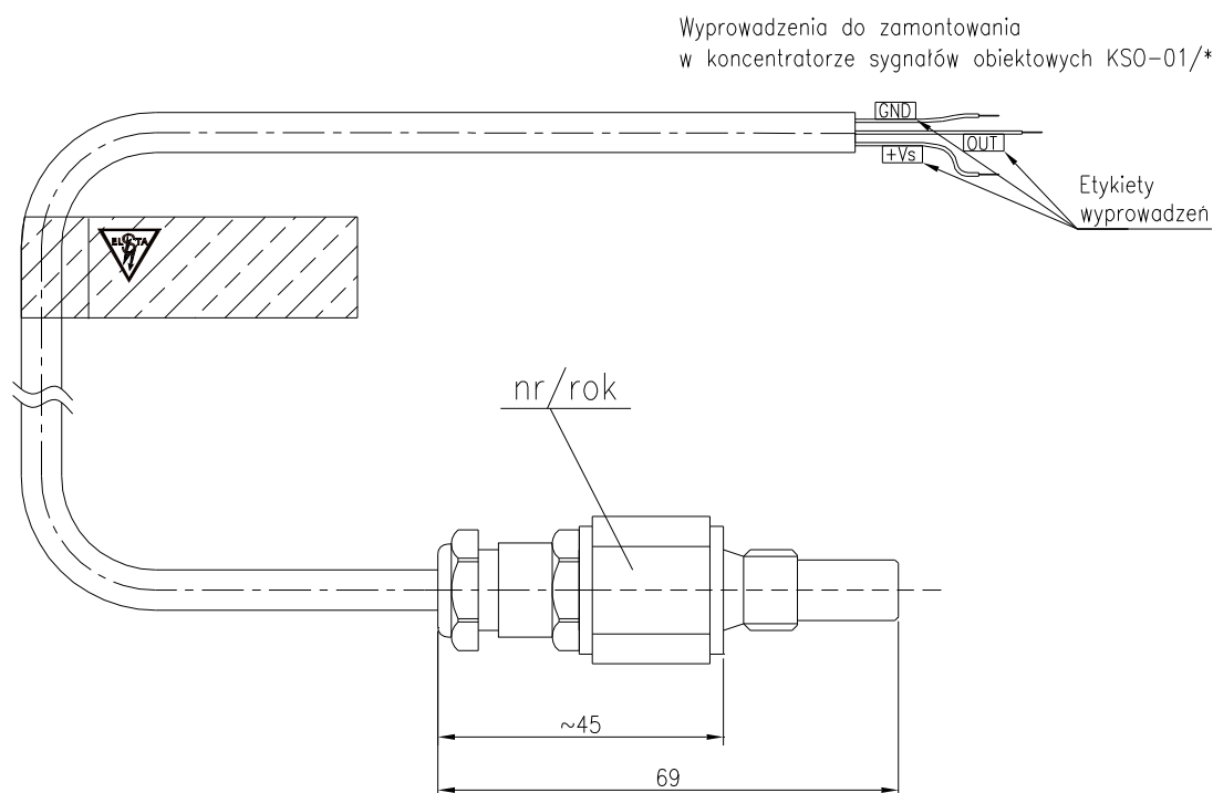
CZUJNIK TEMPERATURY TYPU CZT-03 – rysunek katalogowy
