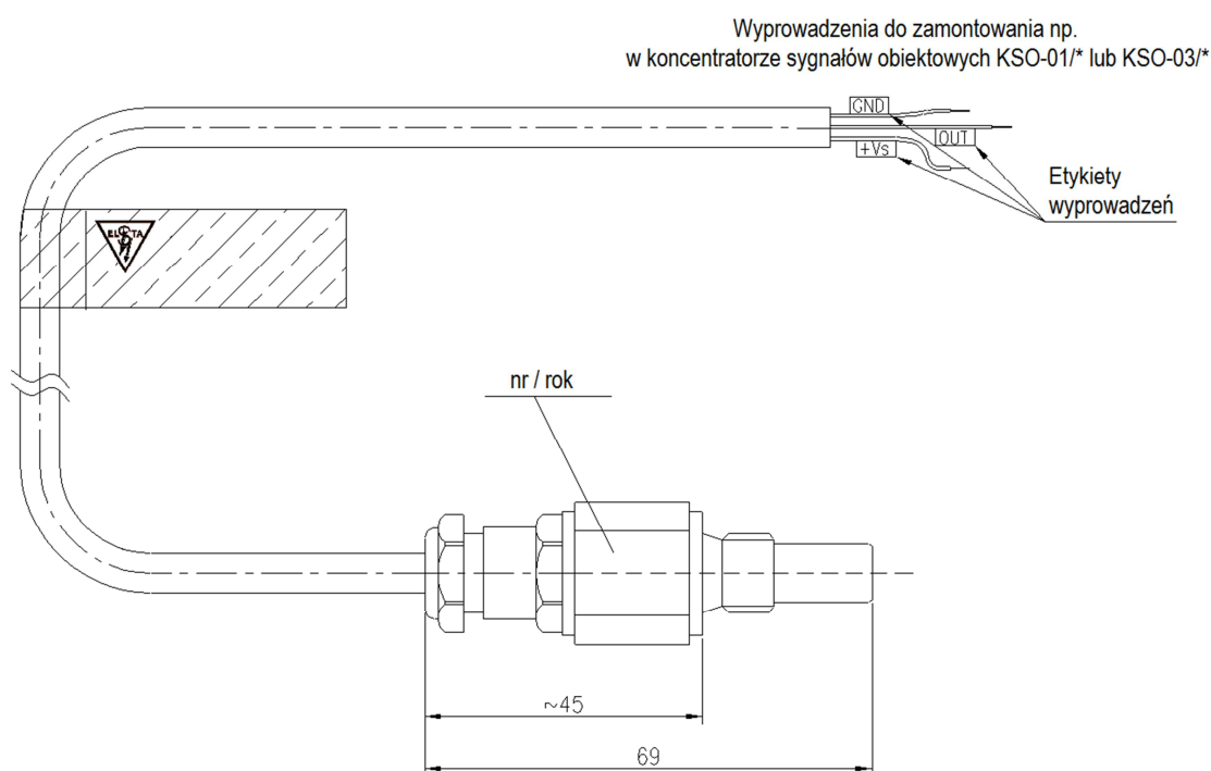
CZUJNIK TEMPERATURY TYPU CZT-01 – rysunek katalogowy
